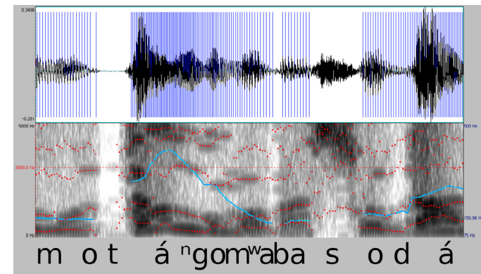
Spektrogramm einer weiblichen Stimme, die Worte in der Sprache Lingala spricht. Gemeinfrei via Wikimedia Commons.
